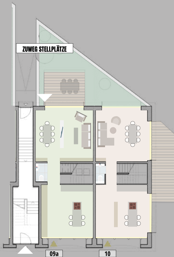
ERDGESCHOSS
